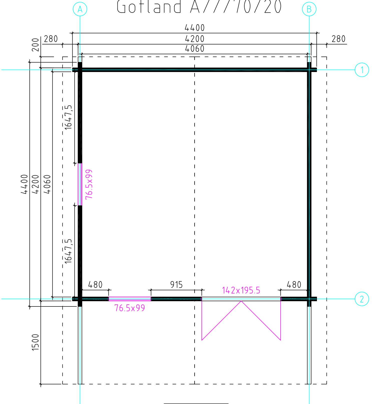
Grundplan
